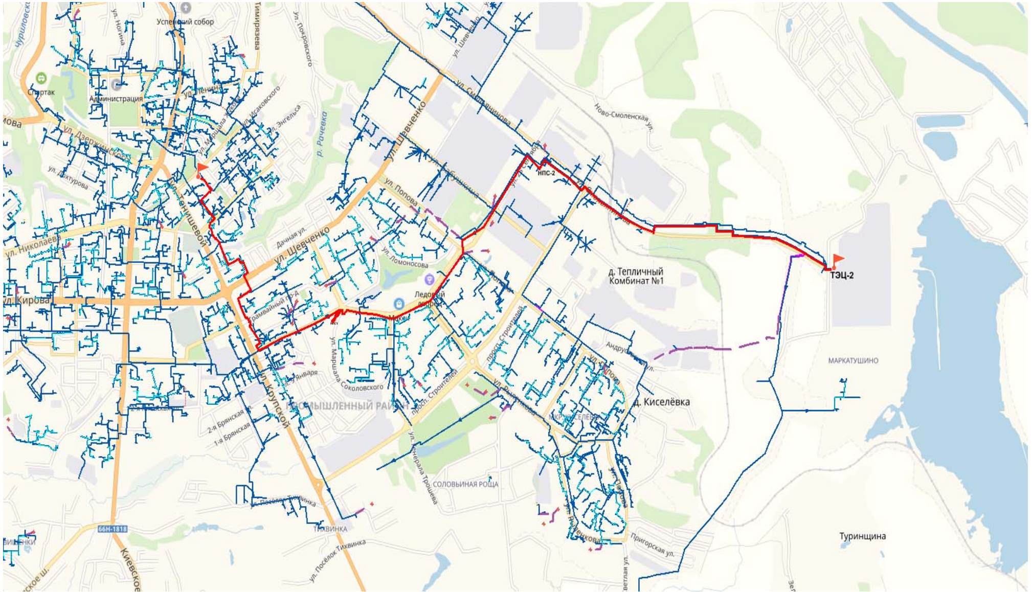
Рисунок 4.1 – Путь пьезометрического графика для участка теплосети от «Смоленской ТЭЦ-2» до перспективной застройки Административное здание с подземной автостоянкой по ул. Исакковского, 8
