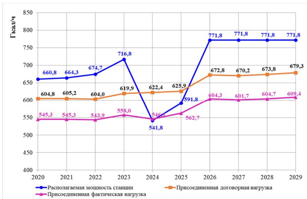
Рисунок 7.1 – График обеспеченности покрытия присоединенных тепловых нагрузок
