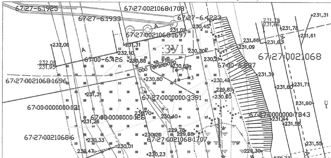
Чертеж размещения объекта на предполагаемых к использованию землях (земельном участке)
